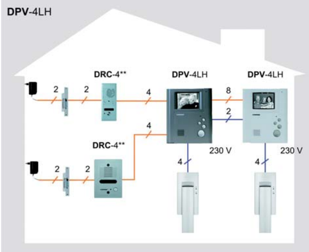
Schemat połączenia DPV-4LH
